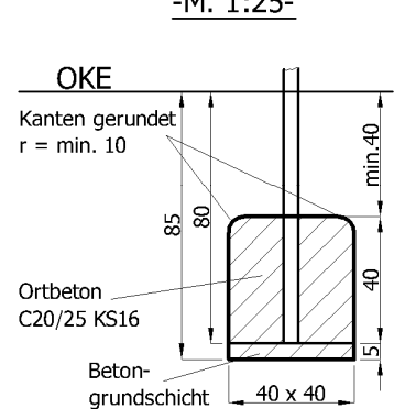
Rutschstangeneinbau -M. 1:25-
